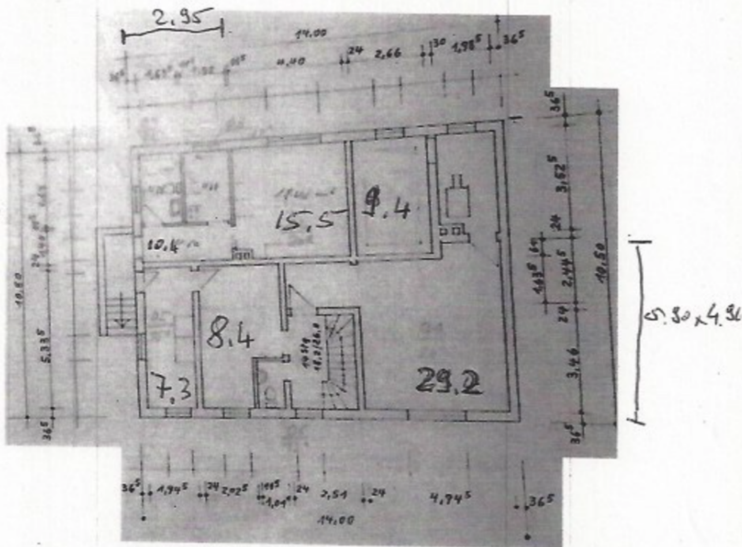
Objekt 2789 606 Kellergeschoss
